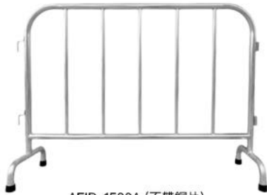
AEIB-1500A (不帶鋼片) 1.5米不銹鋼圍欄 (雙掛鉤) 尺寸: (L) 1500 x (H) 1000mm
