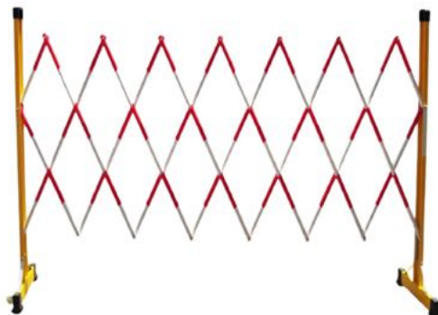
AEBA-001 玻璃纖維伸縮圍欄 尺寸: (H) 1200 x (L) 2500mm 淨重: 約5.5kg
