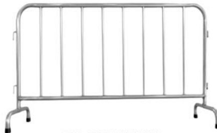
AEIB-2000A (不帶鋼片) 2米不銹鋼圍欄 (雙掛鉤) 尺寸: (L) 2000 x (H) 1000mm
