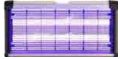
AEMF-40W 紫光滅蚊燈 誘蚊方式: 紫外線誘蚊 應用面積: 20~200 平方米 尺寸: (W) 650 x (D) 55 x (H) 245mm 插電式(放置位置附近需有電位) 功率: 40W (單一燈管20W) 電網電壓: 2500V
