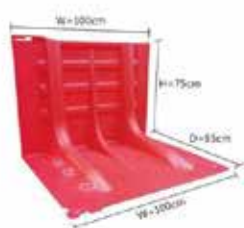
AEBA-015 防洪擋板
