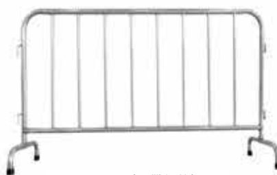
AEIB-2000A (不帶鋼片) 2米不鏽鋼圍欄(雙掛勾) 尺寸: 2000(L) x 1000(H) mm
